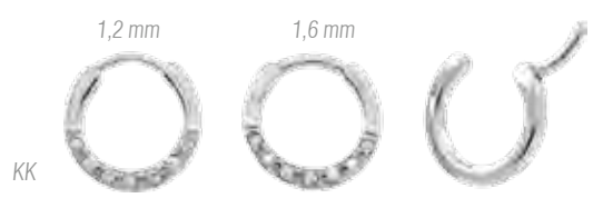
SL270 Chirurgenstahl Clicker rund 7 KRISTALLE Surgical steel clicker round 7 CRYSTALS MEHRERE STÄRKEN | SEVERAL THICKNESSES: 1,2 / 1,6 mm STABLÄNGE | BAR LENGTH: 6 mm – BREITE | WIDTH: 10 mm – HÖHE | HEIGHT: 11 mm
