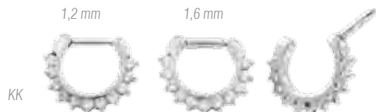
SL266 Chirurgenstahl Clicker 11 KRISTALLE Surgical steel clicker 11 CRYSTALS MEHRERE STÄRKEN | SEVERAL THICKNESSES: 1,2 / 1,6 mm STABLÄNGE | BAR LENGTH: 7 mm – BREITE | WIDTH: 10 mm – HÖHE | HEIGHT: 8 mm
