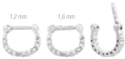
SL278 Chirurgenstahl Clicker 10 KRISTALLE Surgical steel clicker 10 CRYSTALS MEHRERE STÄRKEN | SEVERAL THICKNESSES: 1,2 / 1,6 MM STABLÄNGE | BAR LENGTH: 7 MM — BREITE | WIDTH: 10 MM — HÖHE | HEIGHT: 8 MM
